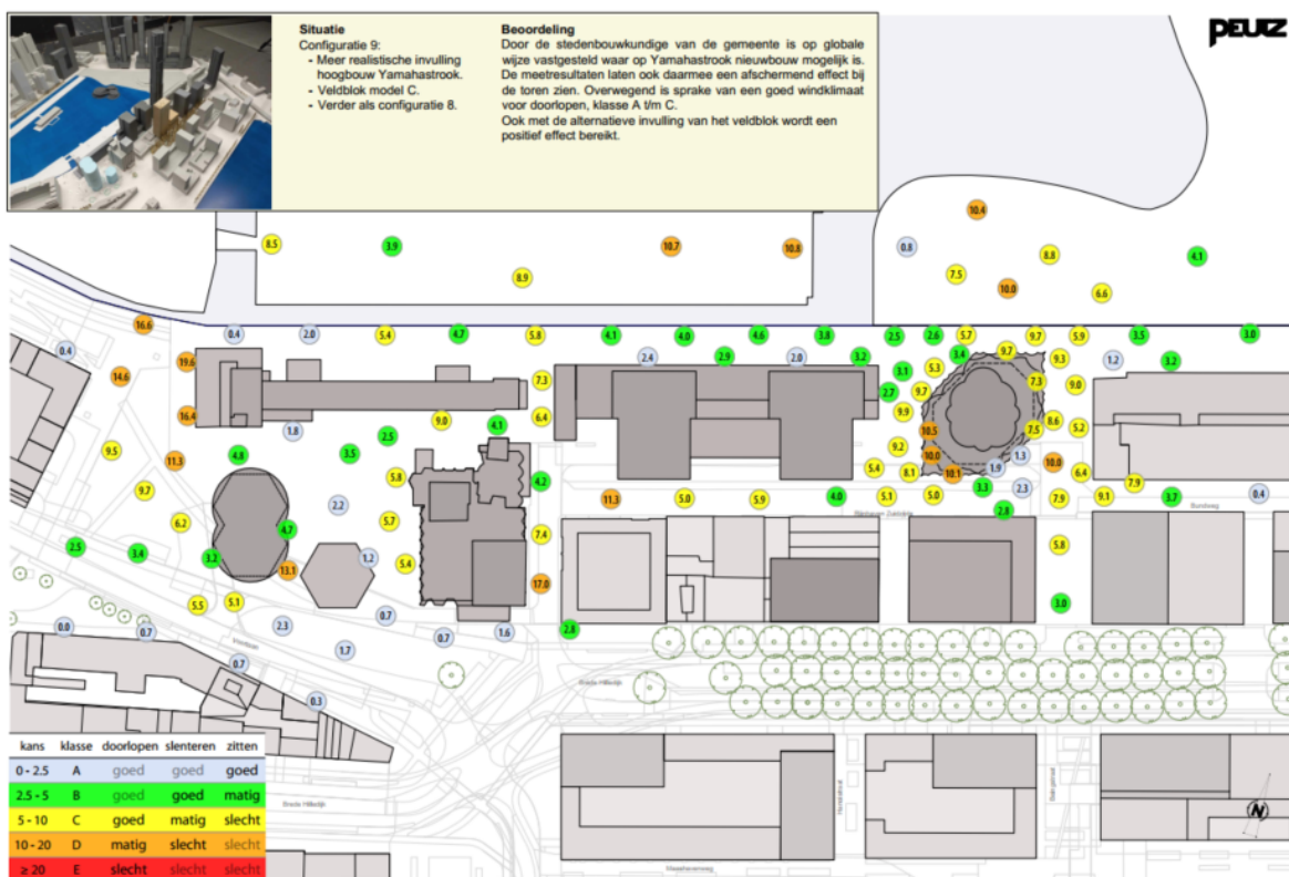
Figuur 6.24: Windklimaat in de meest gunstige onderzoekssituatie (bron: Rapportage Peutz, zie bijlage 12)
