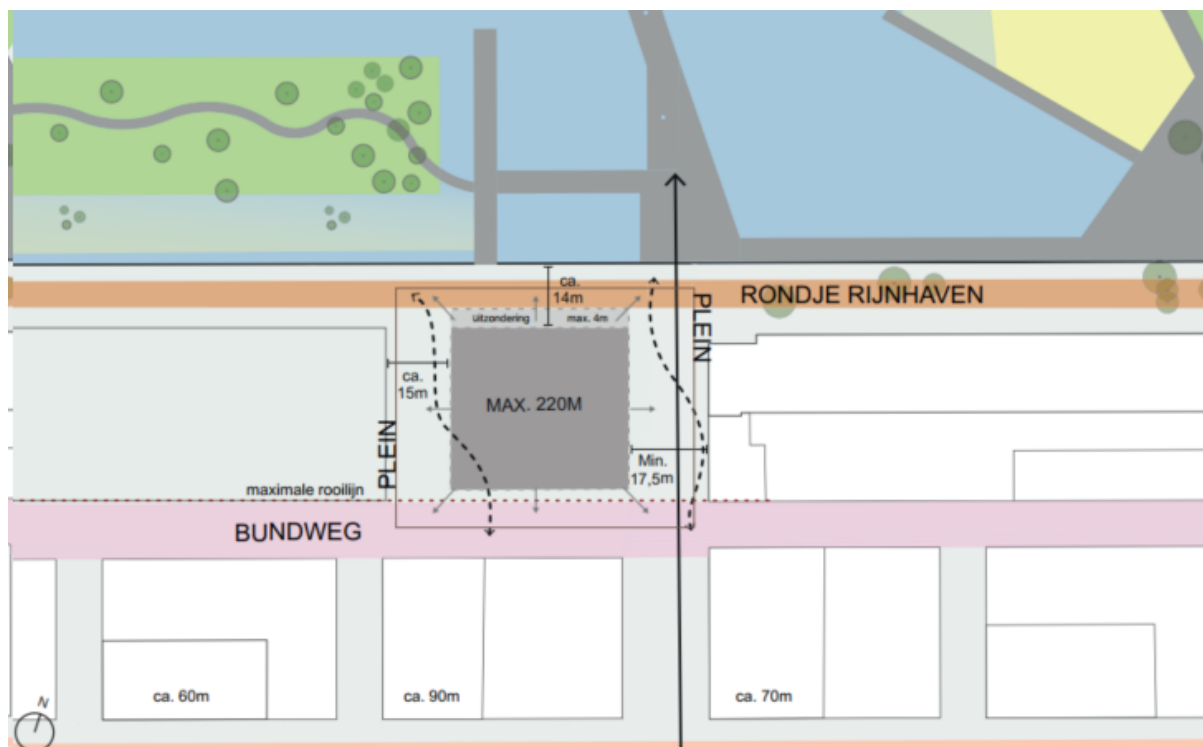
Figuur 2.9: Overzicht toren (bron: Codrico NvU)
