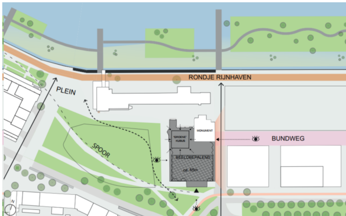
Figuur 2.6: Overzicht beeldbepalend silogebouw (bron: Codrico NvU)
