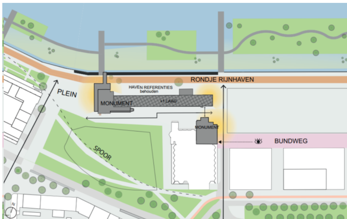
Figuur 2.5: Overzicht monumentaal fabrieksgebouw (bron: Codrico NVU)
