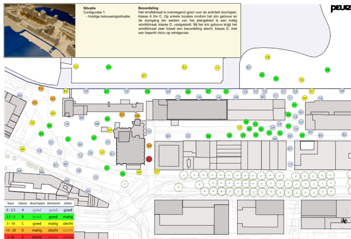
Figuur 6.22: Windklimaat in de huidige situatie (bron: Rapportage Peutz, zie bijlage 12)
